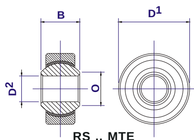
RS .. MTE
