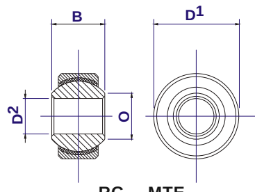
RG .. MTE
